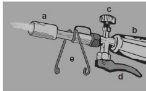
Figura 73 – Maçarico.
