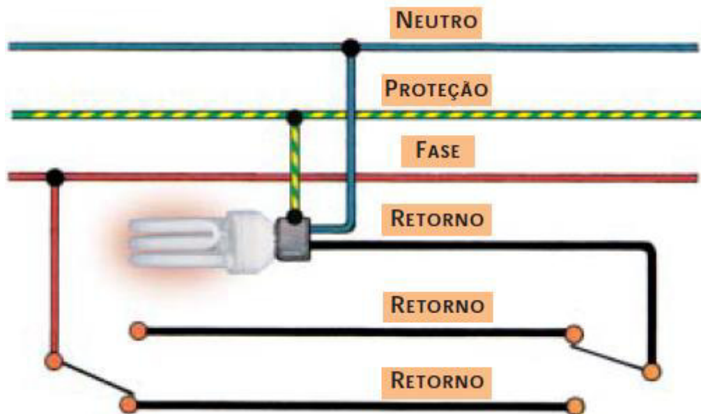
Figura 140 – Esquema equivalente.
