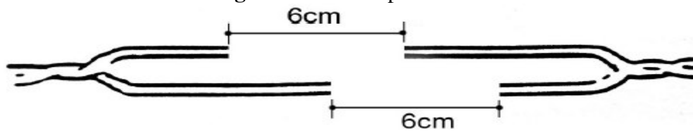
Figura 183 – Decapar o cabo.
