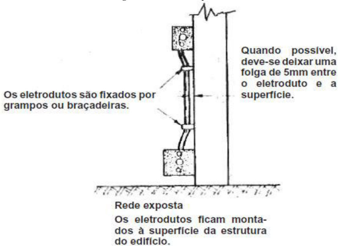
Figura 112 - Rede exposta.
