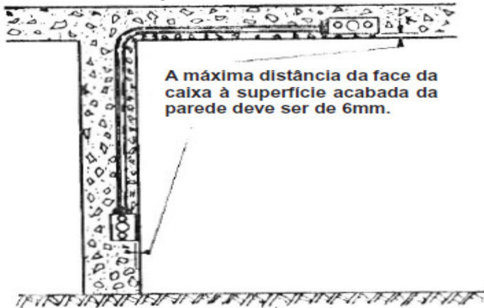
Figura 1099 – Rede embutida.
