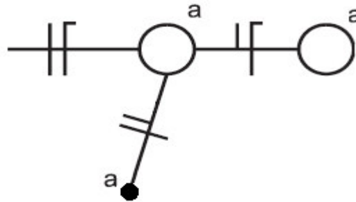
Figura 137 – Esquema unifilar.
