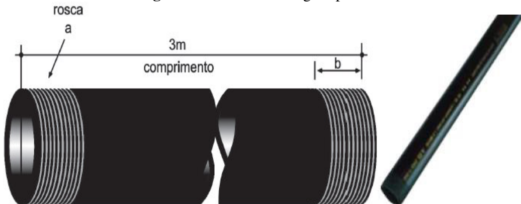
Figura 32 – Eletroduto rígido plástico.
