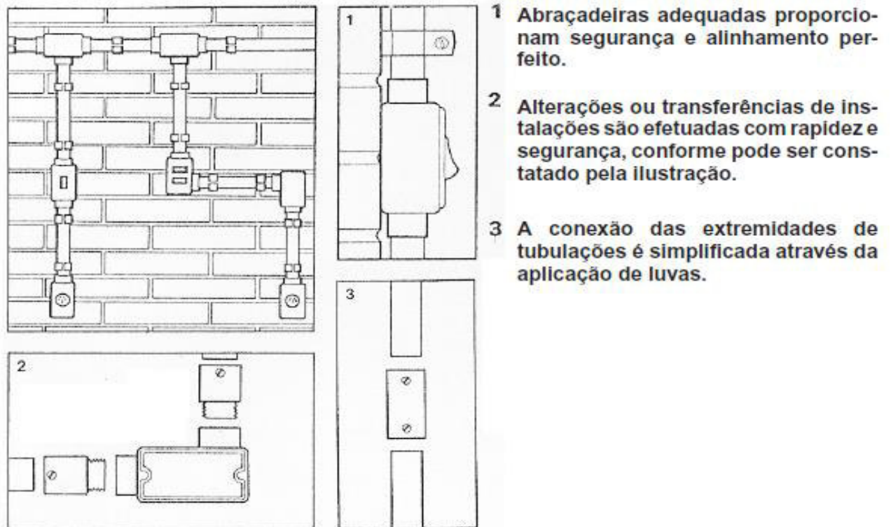
Figura 114 – Conduteles roscável.
