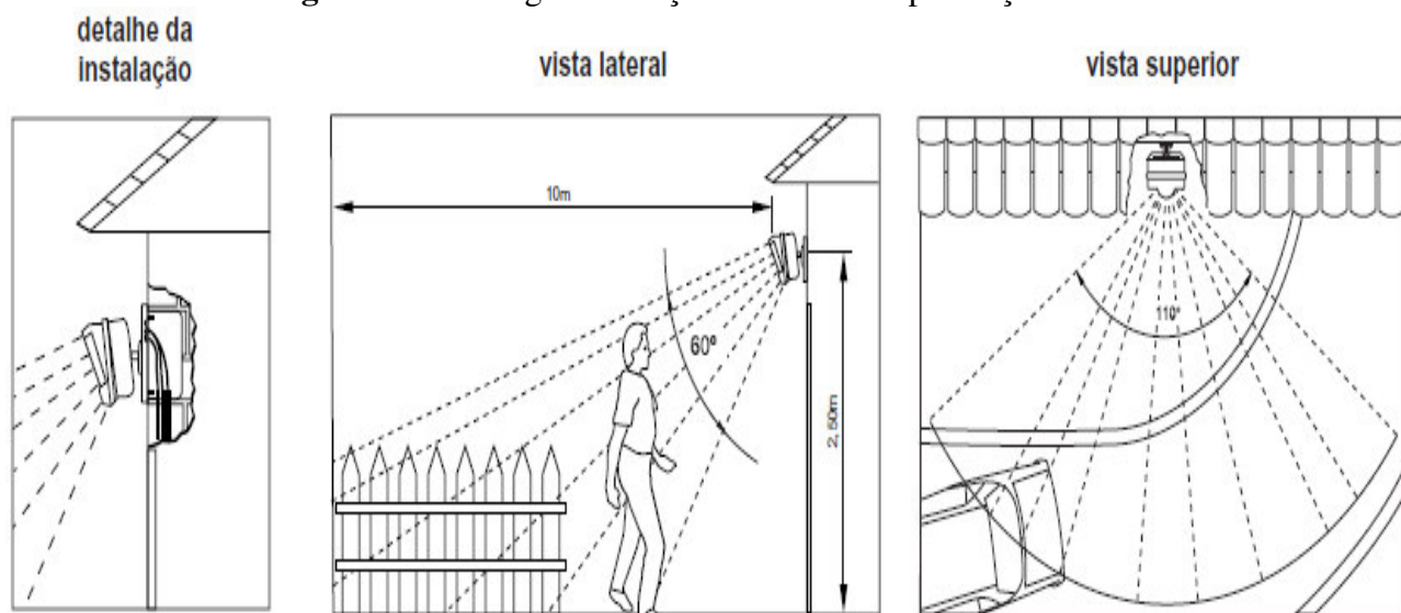
Figura 171 – Range de atuação do sensor de presença.
