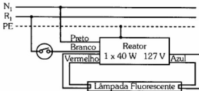
Figura 154 – Esquema multifilar.
