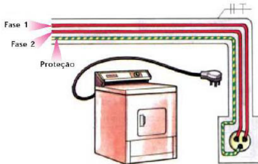
Figura 123 – Tomada bifásica.
