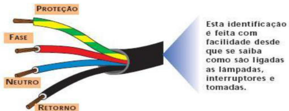
Figura 7 – Padrão de cores.
