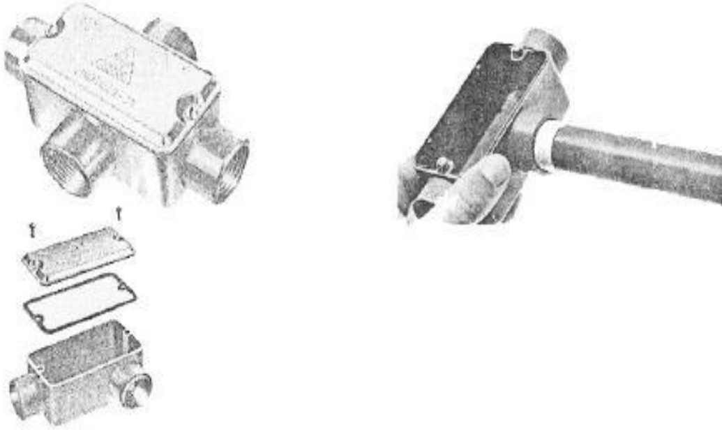
Figura 55 – Conduletes roscáveis.
