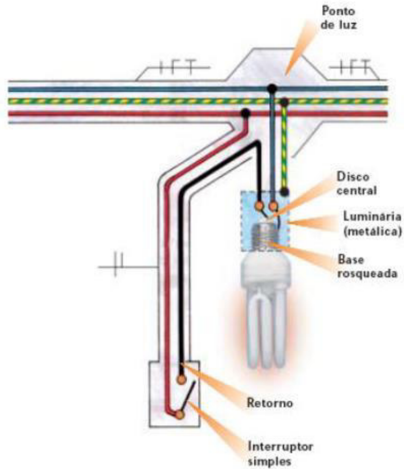
Figura 134 – Esquema de ligação de uma lâmpada com interruptor simples.
