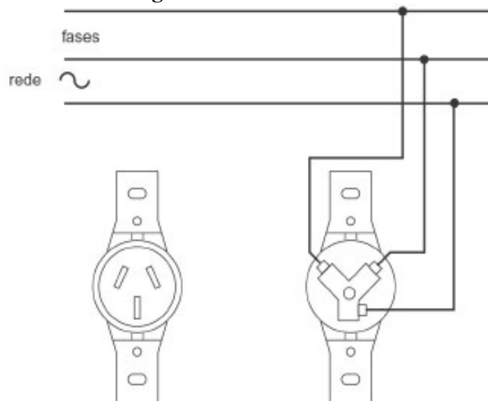
Figura 125 – Tomada 3P.
