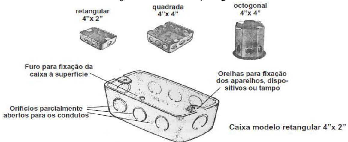
Figura 50 – Caixas de passagem.
